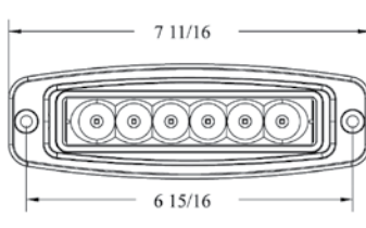
MODEL: LED350
